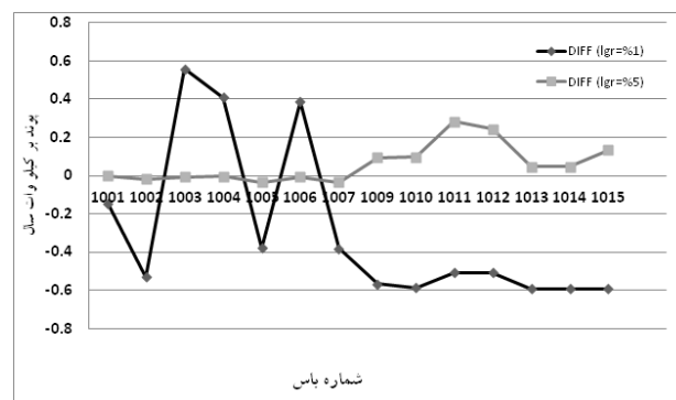
شکل (۸): نمودار اختلاف تعرفه جبران شده جمعی با دو رویکرد افزایشی و نهایی برای دو نرخ رشد بار متفاوت
