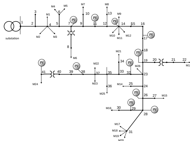
شکل (۲): توپولوژی شبکه آزمایشی ۳۳ شینه IEEE
