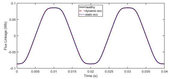
شکل ۳۲: شار پیوندی کل فاز a از موتور دوطرفه بدون شیار در شرایط بی‌باری
