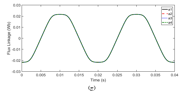
شکل ۳۳: شار پیوندی کلاف‌های مختلف فاز a از موتور دوطرفه بدون شیار در شرایط بی‌باری (الف) شرایط سالم (ب) خطای دینامیک (ج) خطای استاتیک
