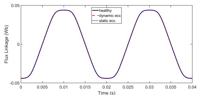
شکل ۱۴: شار پیوندی کل فاز a از موتور یکطرفه بدون شیار در شرایط بی‌باری
