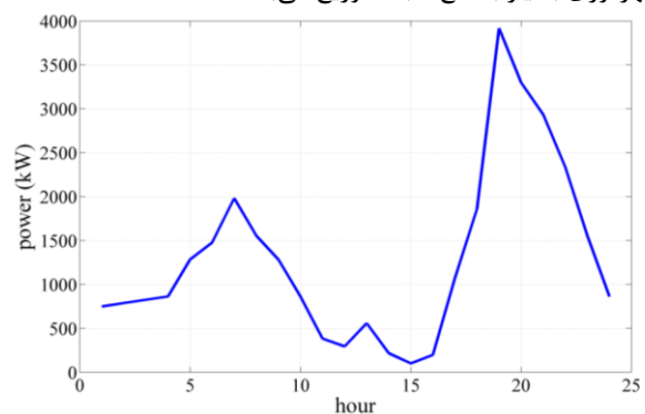
شکل ۷- توان خریداری شده از شبکه بالادست
