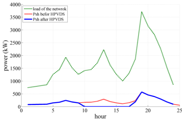
شکل ۸- بار قطع شده در شبکه توزیع در حضور و عدم حضور ریزشبه
