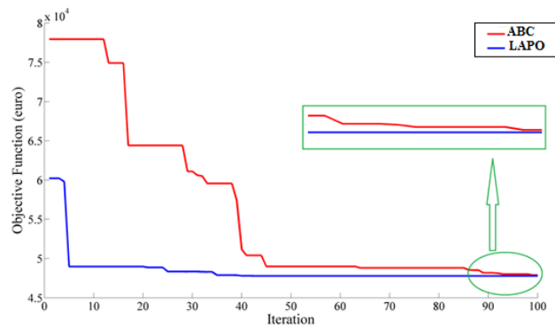
شکل ۵- مقایسه رفتار همگرایی روش‌های مختلف در یافتن بهترین پاسخ برای شبکه ۳۳ باس.
