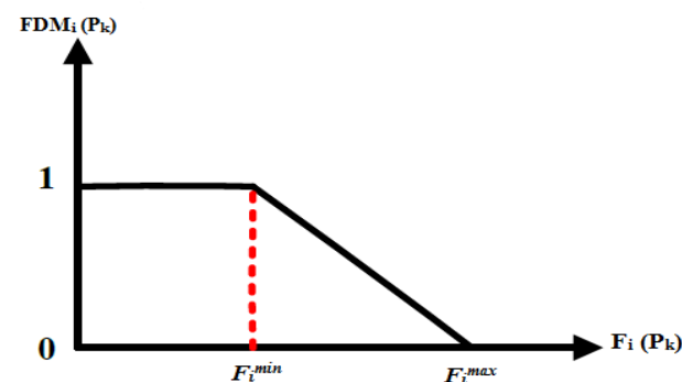
شکل (۳): تابع عضویت متناظر با هدف i
