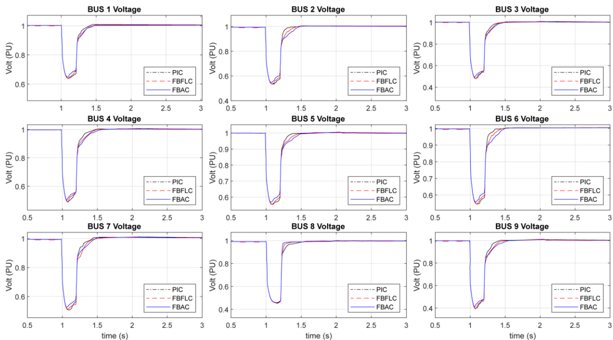
شکل (۱۰): نمودار ولتاژ لحظه‌ای باس‌ها در بازه رخداد خطای به فاز به زمین و پس از حذف آن
