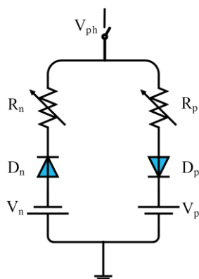
شکل (۲): مدل خطای امپدانس بالا
