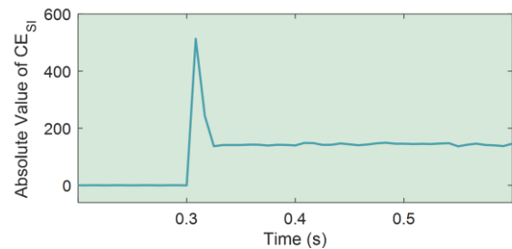
شکل (۶): دامنه سیگنال مؤلفه تحمیلی خطای آنتروپی متقاطع. خطا در 0.3/3 ثانیه رخ داده است.
