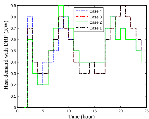
شکل ۱۲- مقایسه تقاضای حرارتی با حضور برنامه پاسخگویی بار
