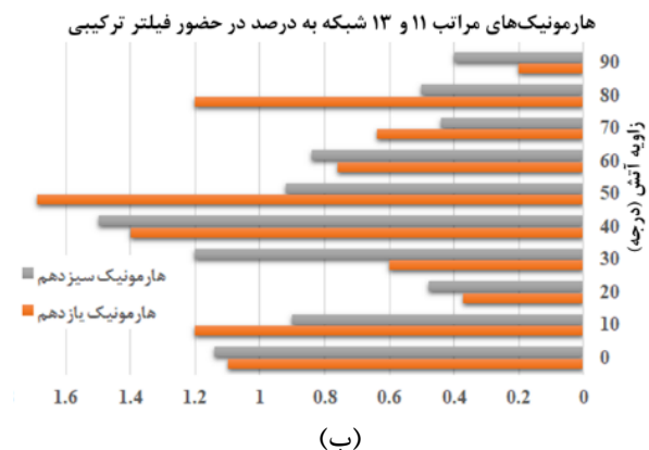
شکل ۱۲: هارمونیک‌های جریان شبکه توزیع با فیلتر ترکیبی: (الف) هارمونیک‌های پنجم و هفتم، (ب) هارمونیک‌های یازدهم و سیزدهم
