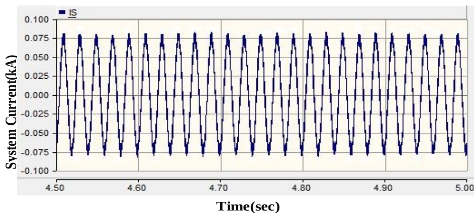
شکل ۱۷: جریان شبکه با فیلتر فعال مبتنی بر CSC با افزایش ۱۰۰ برابری المان‌های پس‌یو
