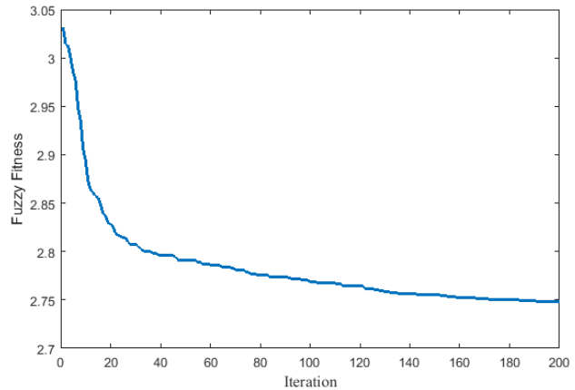
شکل (۶)، نمودار همگرایی الگوریتم ازدحام ذرات در سناریو دوم
