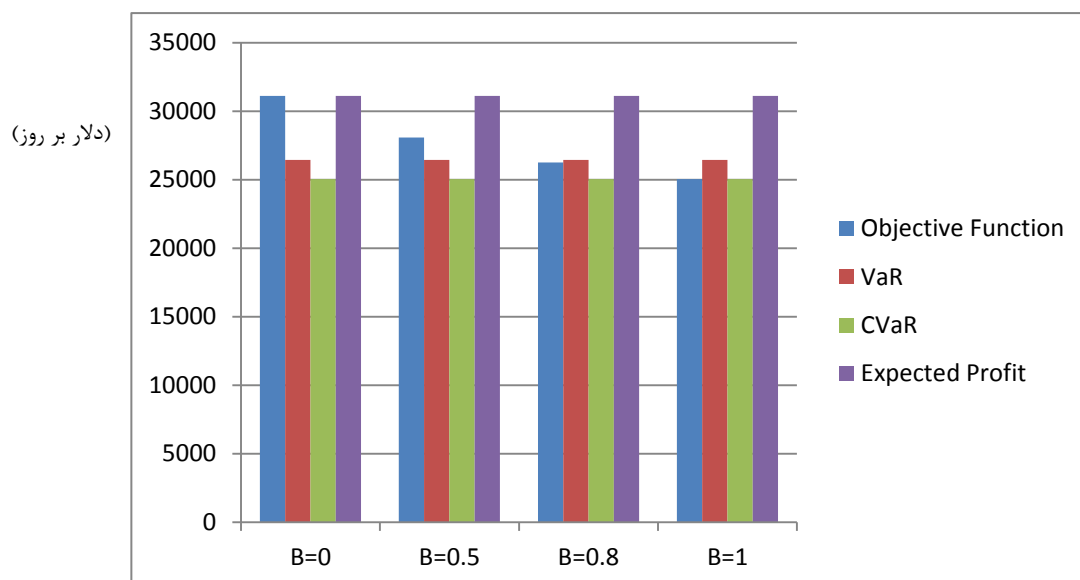
شکل ۶. نمودار میله‌ای شاخص‌های مد نظر خرده‌فروش بازاری مقادیر متفاوت \beta
