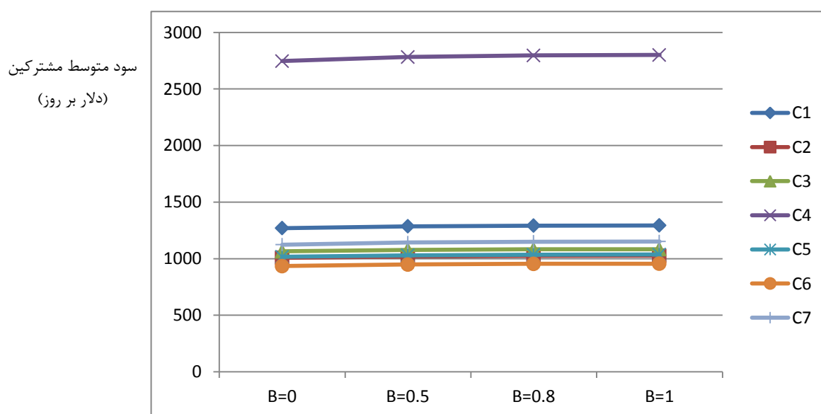
شکل ۷. نمودار مقایسه سود متوسط مشترکین بازاری مقادیر متفاوت \beta
