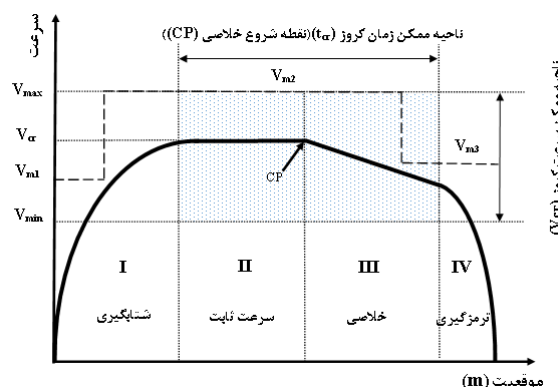
شکل (۱): مشخصه سرعت - مکان (پروفایل سرعت) نمونه با چهار حالت کاری و نواحی ممکن متغیرهای تصمیم
