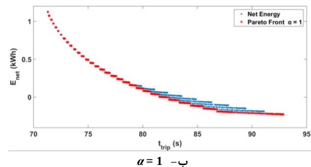
شکل (۴): گراف انرژی-زمان همراه با جبهه پرتو برای یک فاصله بین ایستگاهی سراسیبی نمونه با مقادیر مختلف \alpha
