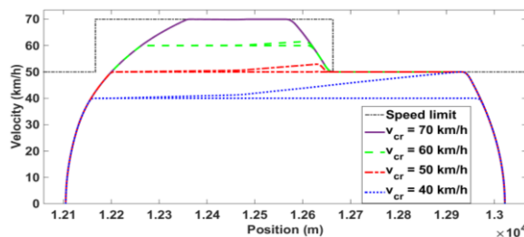
شکل (۲): مشخصه‌های سرعت برای یک فاصله بین ایستگاهی سراسیابی نمونه با مقادیر مختلف پارامترهای تصمیم
