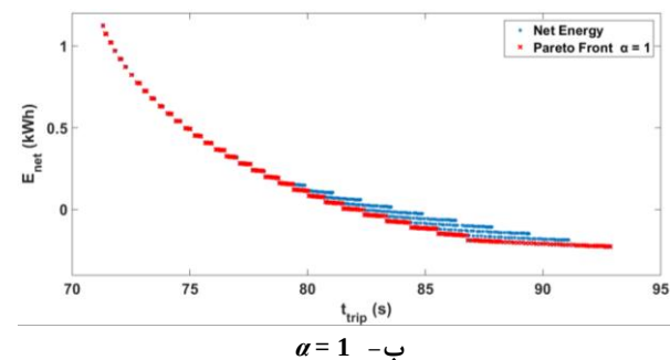
شکل (۴): گراف انرژی-زمان همراه با جبهه پرتو برای یک فاصله بین ایستگاهی سراسیابی نمونه با مقادیر مختلف \alpha
