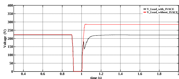
شکل ۱۸: ولتاژ بار 10kW در حالت اتصال سیم گارد به زمین و بار کامل
