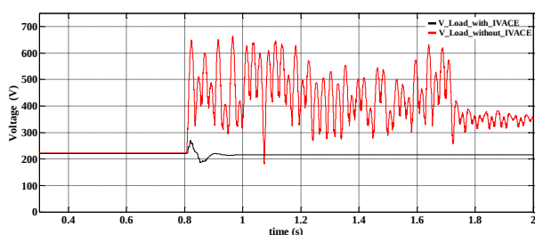
شکل ۲۰: ولتاژ ورودی سایت مخابراتی در زمان خارج شدن بار 10kW
