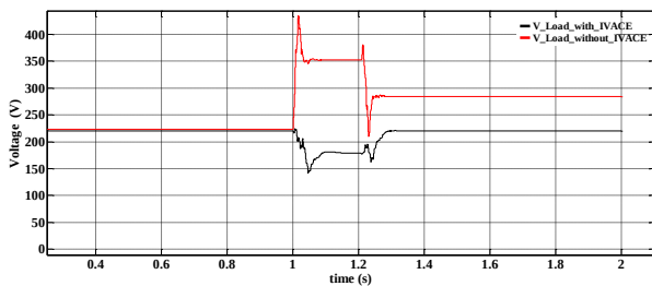
شکل ۱۵: ولتاژ بار 10KW در حالت اتصال کوتاه تک فاز بر روی خط انتقال هوایی
