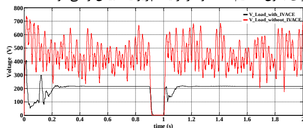
شکل ۱۷: ولتاژ ورودی سایت مخابراتی در حالت اتصال سیم گارد به زمین و بی‌باری
