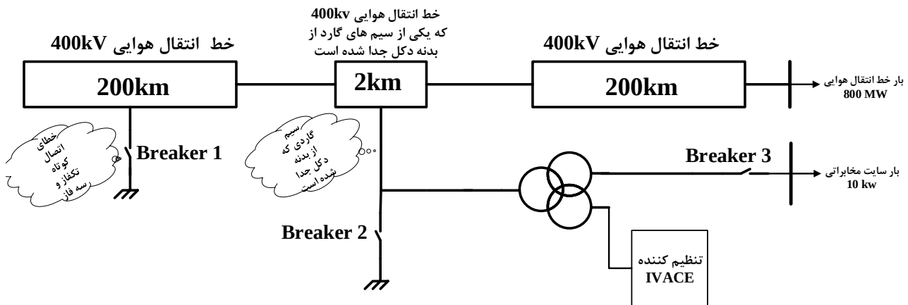
شکل ۱۳: مدار کلید زنی شبکه
