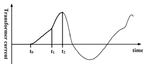
شکل (۲): نمونه ای از جریان هجومی
