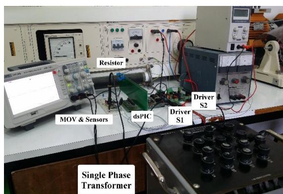
شکل (۴): نمونه آزمایشگاهی اولیه SSICL
