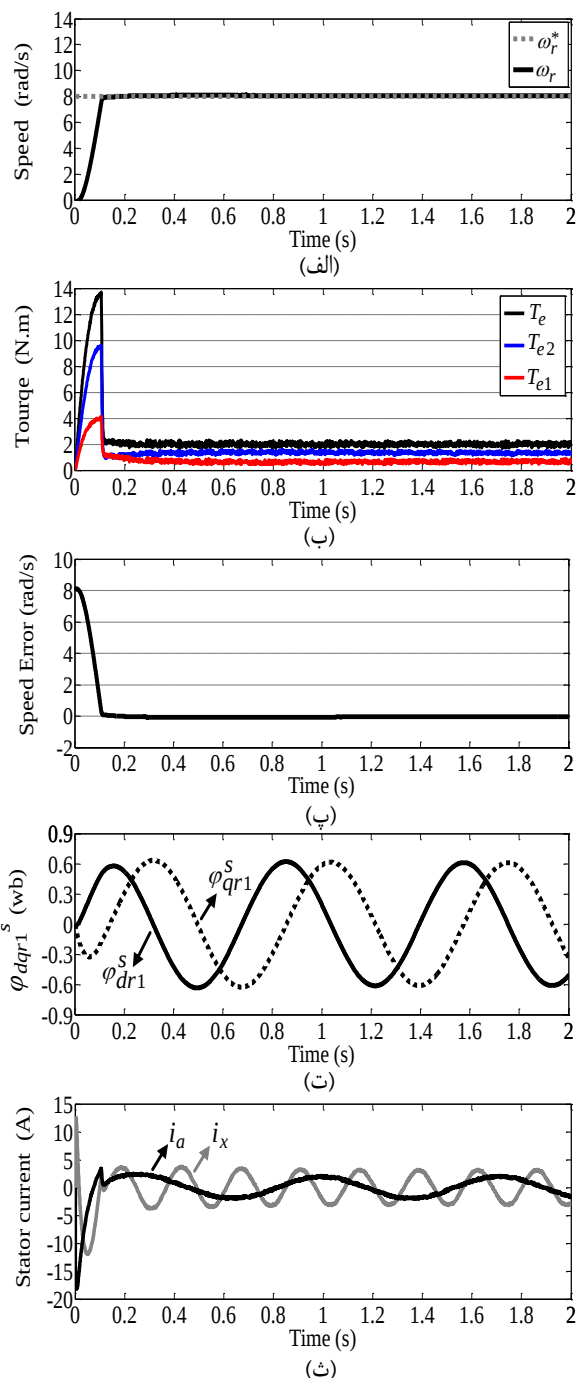
شکل (۱۴): نتایج شبیه‌سازی روش پیشنهادی در پاسخ به فرمان سرعت 8 \text{ rad/s} و گشتاور 2 \text{ N.m} : (الف) پروفایل سرعت روتور، (ب) پروفایل گشتاور، (پ) خطای سرعت، (ت) مؤلفه‌های q و d شار روتور در سیم‌پیچ abc روی محورهای d^s - q^s و (ث) جریان فاز a سیم‌پیچ abc و جریان فاز اول (x) سیم‌پیچ xyz.
