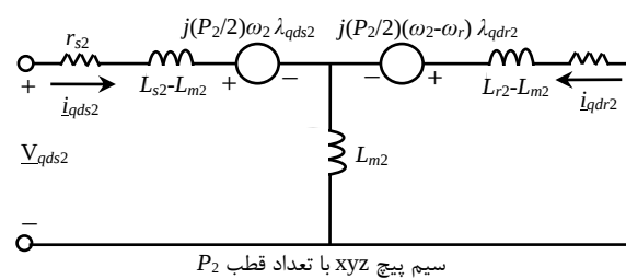
شکل (۳): مدار معادل d-q ی DSWIM [5].
