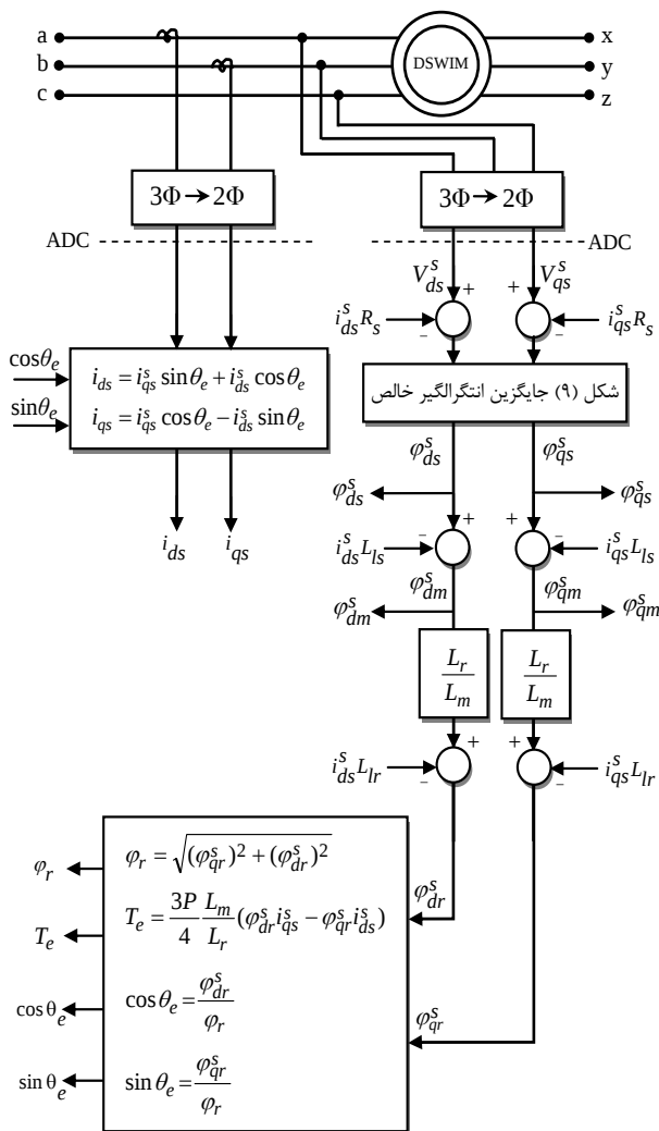
شکل (۸): نمایش شماتیکی تخمین سیگنال‌های برگشتی مدل ولتاژ برای سیم‌پیچ abc در درایو DSIM.
