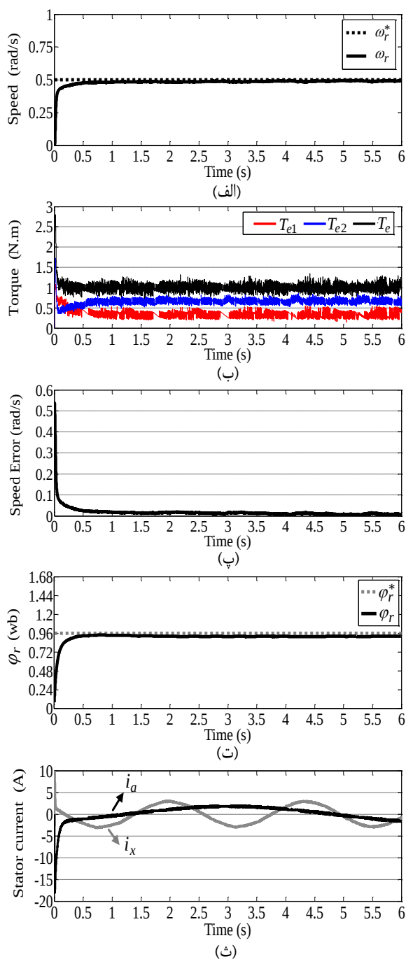
شکل (۱۳): نتایج شبیه‌سازی روش پیشنهادی در پاسخ به فرمان سرعت 0.5 \text{ rad/s} و گشتاور 1 \text{ N.m} : (الف) پروفایل سرعت روتور، (ب) پروفایل گشتاور، (پ) خطای سرعت، (ت) شار روتور و (ث) جریان فاز a سیم‌پیچ abc و جریان فاز اول (x) سیم‌پیچ xyz.
