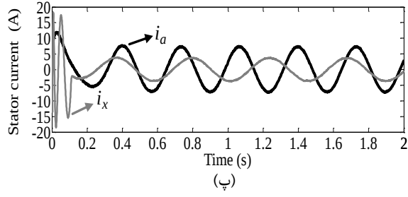
شکل (۱۴): نتایج شبیه‌سازی روش مرسوم در پاسخ به فرمان سرعت 8 \text{ rad/s} و گشتاور 2 \text{ N.m} : (الف) پرو فایل سرعت روتور، (ب) پرو فایل گشتاور، (پ) جریان فاز a سیم‌پیچ abc و جریان فاز اول (x) سیم‌پیچ .xyz
