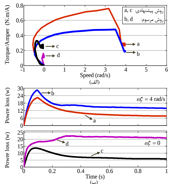
شکل (۱۸): نتایج شبیه‌سازی روش پیشنهادی و مرسوم در پاسخ به فرمان سرعت صفر با گشتاور ۳ N.m و سرعت ۴ rad/s با گشتاور ۵ N.m (الف) نسبت گشتاور بر آمپر و (ب) مجموع کل تلفات توان (هدایتی و کلیدزنی) در واحدهای اینورتر.
