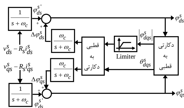
شکل (۹): نمایش شماتیکی الگوریتم پیشنهادی [25] برای حل مشکل آفست DC در درایو DSIM.
