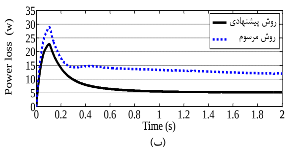
شکل (۱۶): نتایج شبیه‌سازی روش پیشنهادی و مرسوم در پاسخ به فرمان سرعت 8 \text{ rad/s} و گشتاور 2 \text{ N.m} : (الف) نسبت گشتاور بر آمپر (ب) مجموع کل تلفات توان (هدایتی و کلیدزنی) در واحدهای اینورتر.
