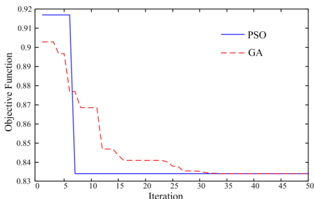
شکل ۳: نمودار همگرایی الگوریتم‌های هوشمند در مثال اول
