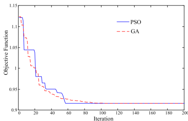
شکل ۴: نمودار همگرایی الگوریتم‌های هوشمند در مثال سوم
