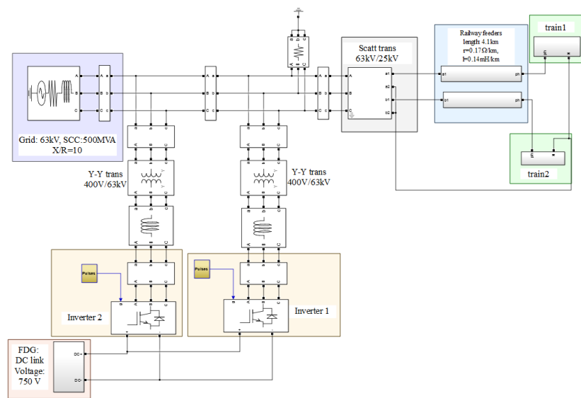
شکل (۱): نمای سیستم تغذیه قطار توسط شبکه و تولید پراکنده انعطاف پذیر اتصال یافته توسط اینورتر دابل
