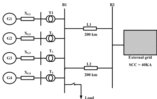
شکل (۱۰): سیستم مورد مطالعه
