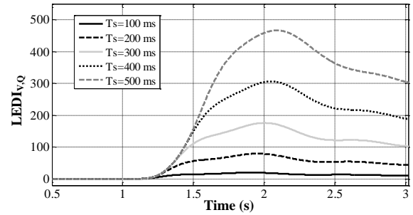
شکل (۱۲): تأثیر افزایش T_s بر LEDI
