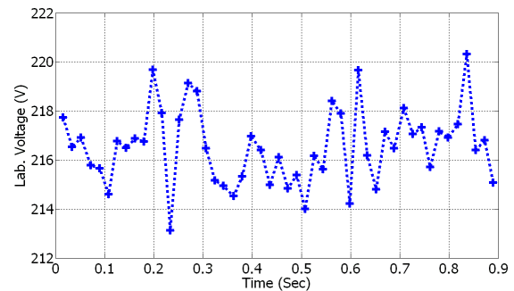
شکل (۱۹): دامنه و تغییرات ولتاژ آزمایشگاه در هنگام آزمایش
