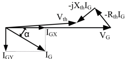
شکل (۶): دیاگرام فازوری پارامترهای ترمینال ژنراتور
