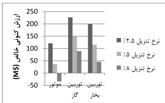
شکل (۱۷) تأثیر نرخ تنزیل بر ارزش کنونی خالص
