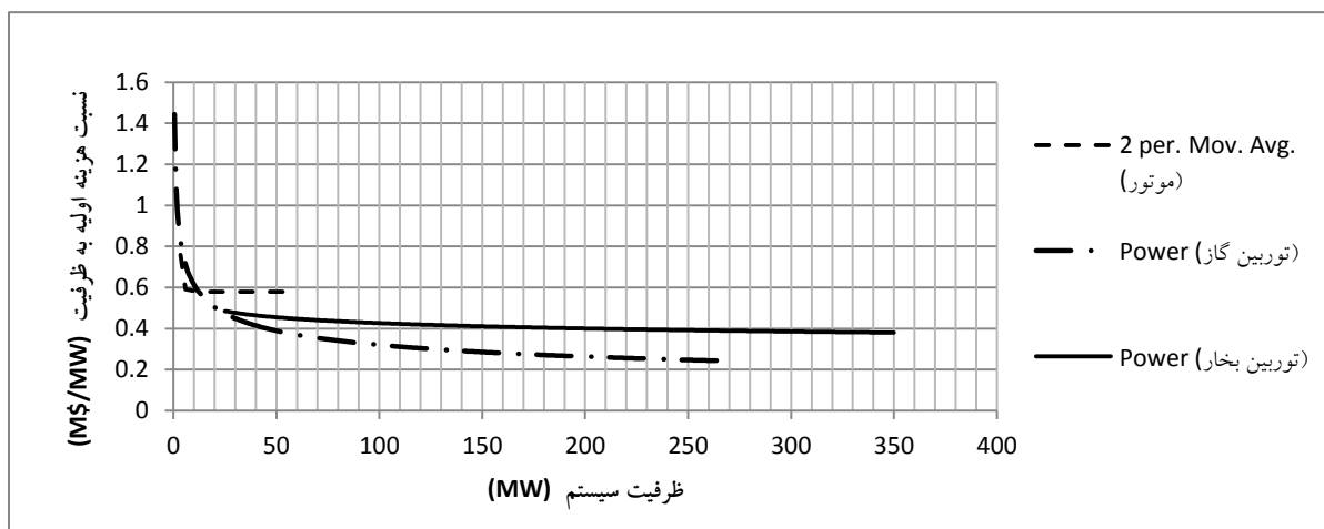
شکل (۸) تغییرات نسبت هزینه اولیه به ظرفیت با ظرفیت سیستم
