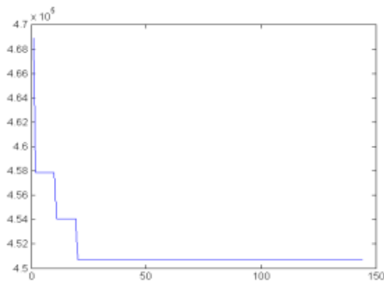
شکل (۵): نمودار هزینه کلی سیستم با در نظر گرفتن قیود امنیتی
