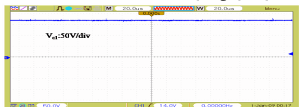
(V C1 )
