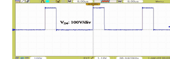
( V_{D4} )
