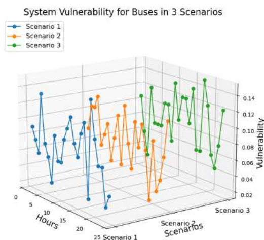
شکل (۵): شاخص آسیب‌پذیری باسباهای سیستم چند منطقه‌ای به ازای سه سناریو مختلف برای ۲۴ یک افق ۲۴ ساعته
