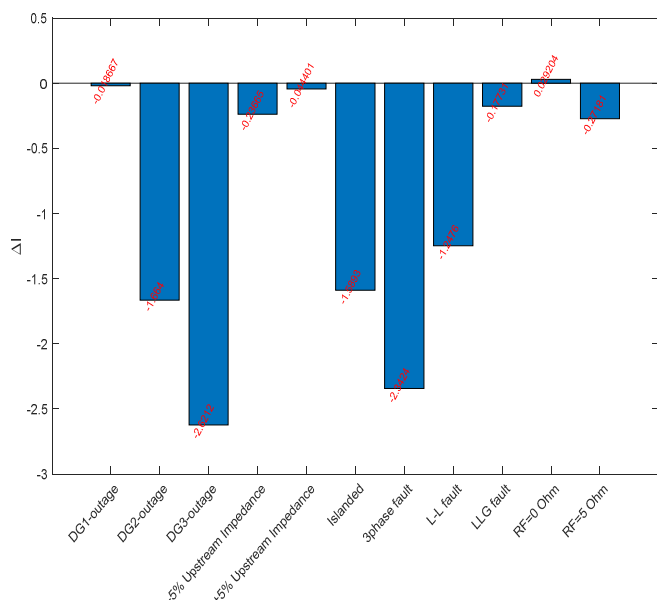
شکل (۹): نتایج محاسبه شاخص سوم برای جریان اندازه‌گیری شده در محل زوج رله اصلی و پشتیبان R15 و R13 ریزشبه تحت مطالعه
