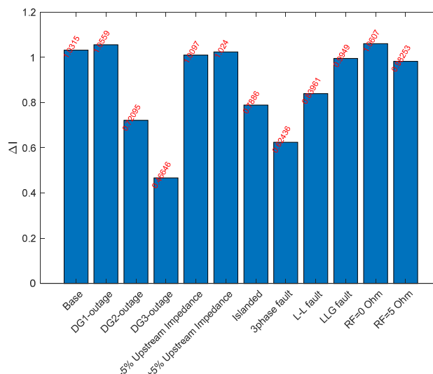
شکل (۸): نتایج محاسبه شاخص دوم برای جریان اندازه‌گیری شده در محل زوج رله اصلی و پشتیبان R15 و R13 ریزشبه تحت مطالعه
