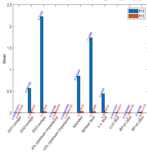
شکل (۷): نتایج محاسبه شاخص MSE برای جریان اندازه‌گیری شده در محل رله‌های اصلی و پشتیبان R15 و R13 ریزشبه تحت مطالعه
