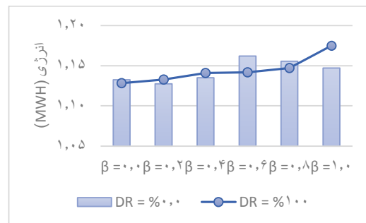
شکل ۷: مقایسه میانگین انرژی ذخیره شده در ذخیره‌ساز به ازای مقادیر مختلف \beta برای دو حالت عدم عرضه و عرضه حداکثر خدمات بارهای پاسخگو در بازار میان‌روزی.
