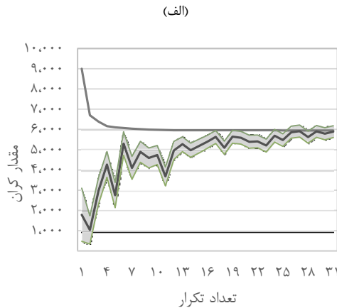
شکل ۳: روند همگرایی کُران‌های بالا و پایین در الگوریتم SDDP برای دو حالت مختلف از میزان مشارکت تجمیع‌گران در بازار IDRX. (الف) بدون امکان مبادله‌ی DR. (ب) مقدار DR ارائه شده در بازار ۱۰۰٪ ظرفیت.
