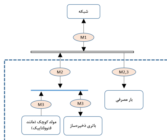
شکل ۳. آرایش‌های مختلف قرارگیری کنتور برای مشترکین کوچک
