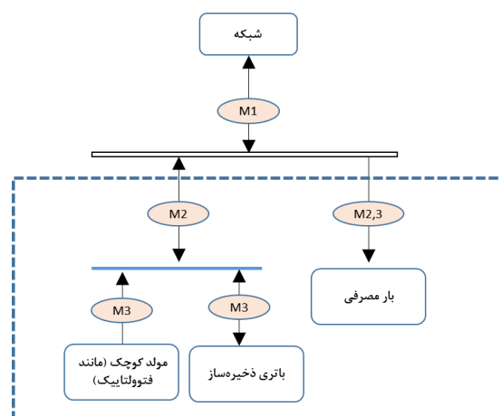
شکل ۳. آرایش‌های مختلف فرارگیری کنتور برای مشترکین کوچک
