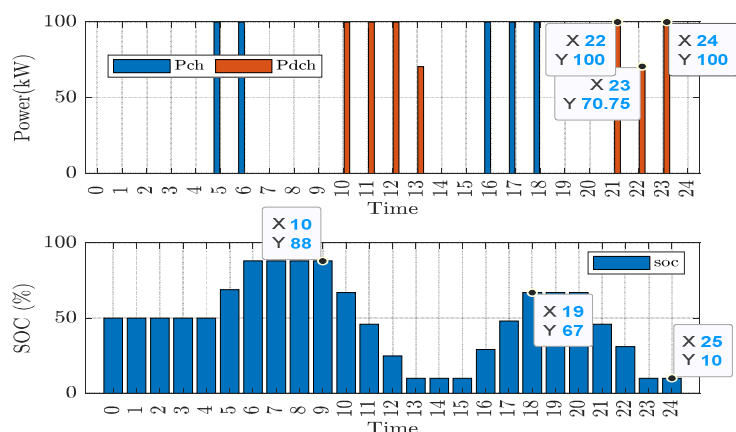
شکل ۱۱ برنامه‌ریزی شارژ و دشارژ MESS شماره ۳
