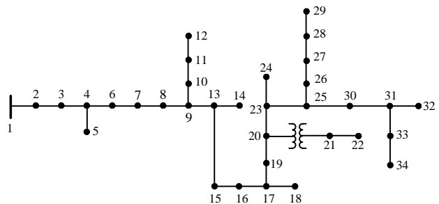
شکل (۷): شبکه تست اصلاح شده IEEE-34 Node
