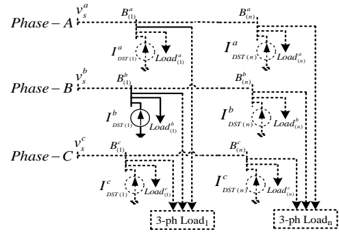
شکل (۱): شبکه نمونه توزیع شعاعی فشار ضعیف
