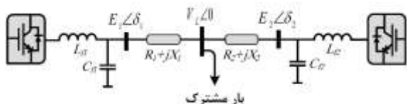
شکل (۱): نمودار تک خطی یک ریزشبکه‌ی جزیره‌ای
