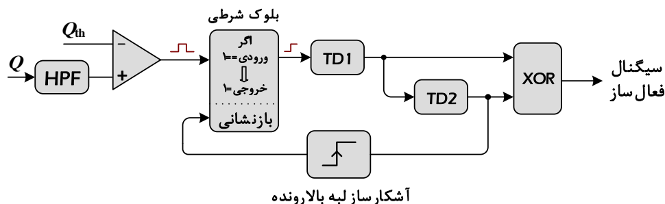
شکل (۵): ساختار واحد تولیدکننده‌ی سیگنال فرمان آغاز فرآیند اصلاح مشخصه‌افتی
