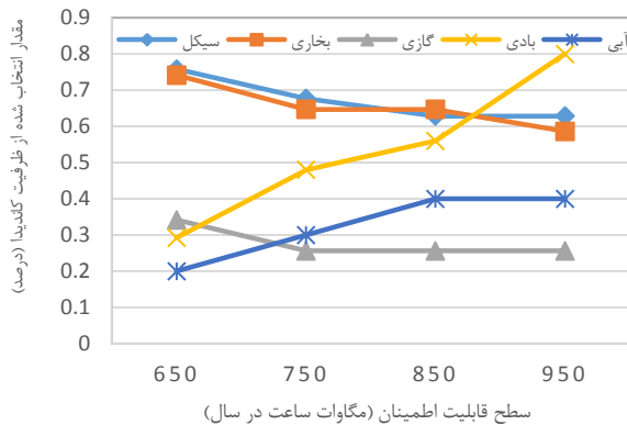
شکل (۲): کاهش هزینه کل توسعه سیستم تولید و کاهش هزینه آلودگی با مشارکت مزارع بادی
