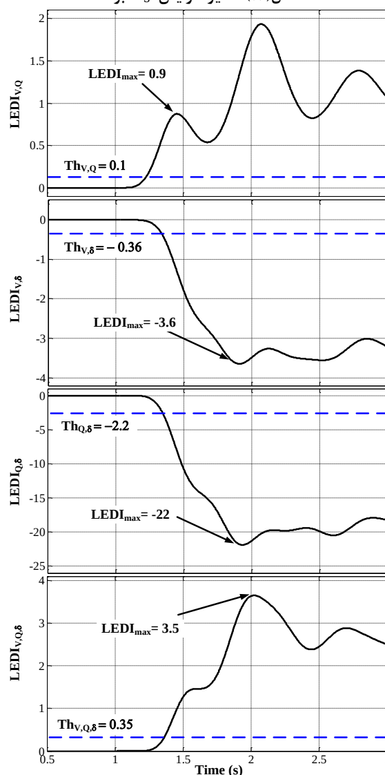
شکل (۱۳): تغییرات LEDI‌های معرفی‌شده به ازای بدترین شرایط ممکن برای تعیین مقادیر آستانه (Th)
