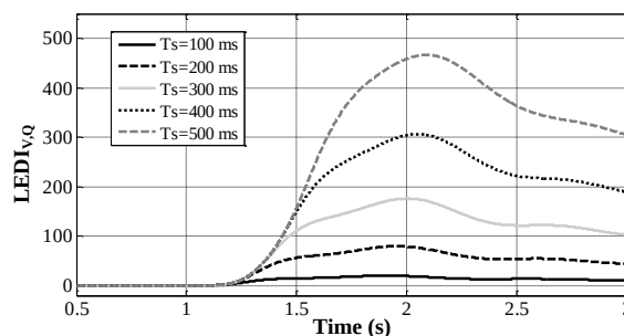
شکل (۱۲): تأثیر افزایش T_s بر LEDI
