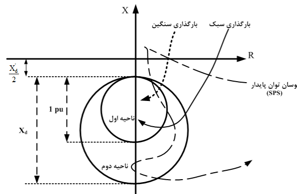
شکل (۱): مشخصه‌ی عملکردی رله‌ی LOE و مکان هندسی تغییرات امپدانس در شرایط مختلف
