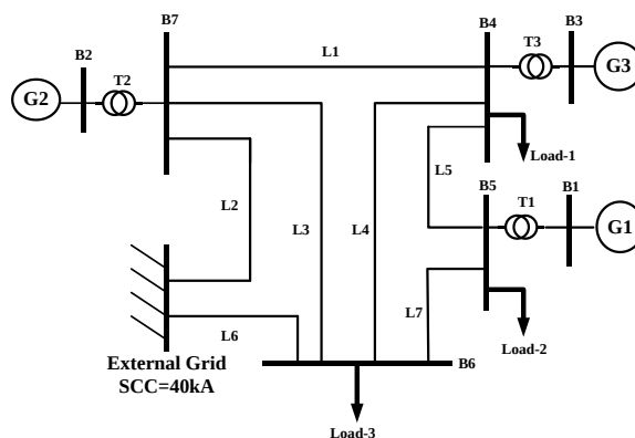
شکل (۱۵): سیستم سه ماشین مورد مطالعه
