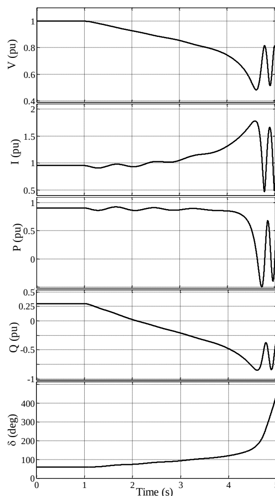
شکل (۳): تغییر کمیت‌های الکتریکی ژنراتور بعد از وقوع LOE
