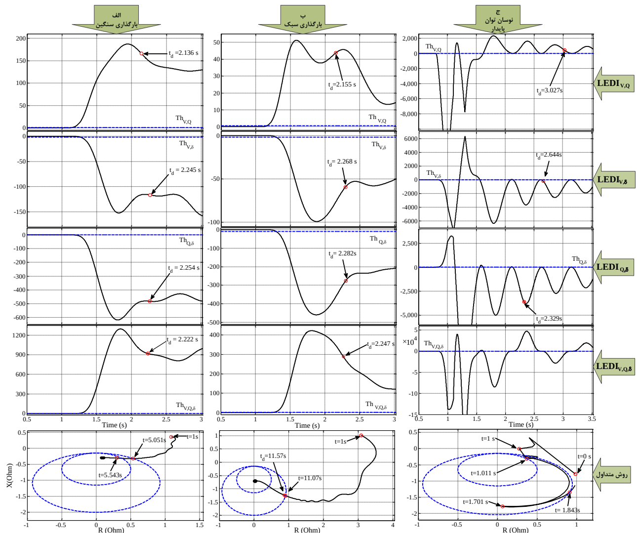
شکل (۱۴): عملکرد LEDI در مقایسه با طرح متداول امپدانسی به ازای وقوع LOE در بارگذاری‌های سنگین (الف) و سبک (ب) و در شرایط نوسان توان پایدار (ج)
