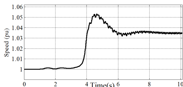
شکل (۴): تغییرات سرعت ژنراتور بعد از وقوع LOE
