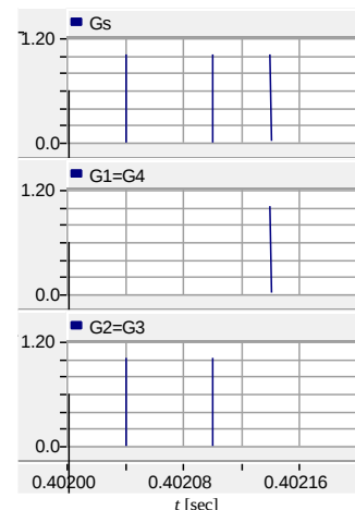
شکل ۲۰- تولید سیگنال‌های کنترل PWM با استفاده از روش فرکانس بالا
