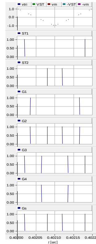
شکل ۱۷: تولید سیگنال‌های کنترل PWM برای S-ZSI با استفاده از روش PWM مدولاسیون سینوسی
