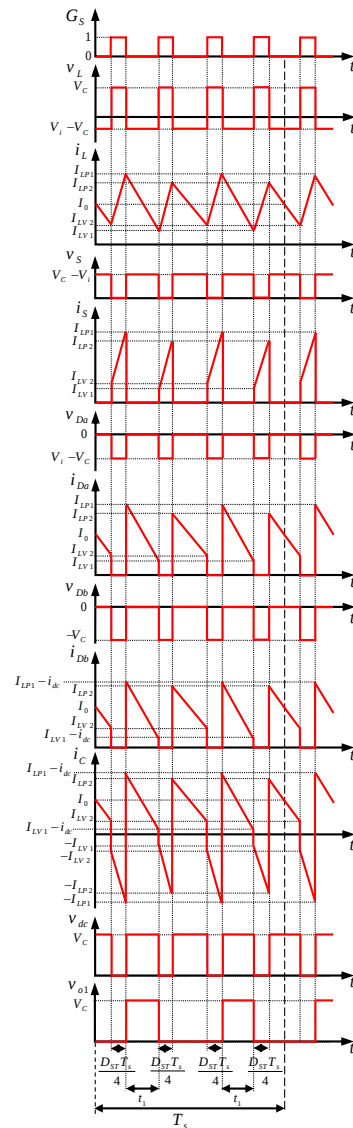
شکل ۷- شکل موج‌های حالت دائمی ولتاژ و جریان اجزای S-ZSI با استفاده از روش اول
