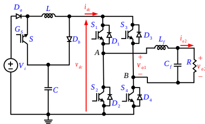
شکل ۲- ساختار S-ZSI
